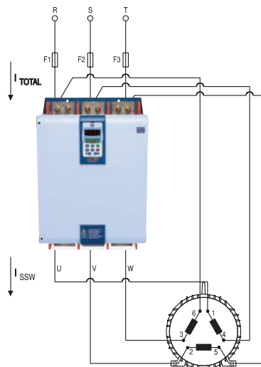
SSW-06内接
