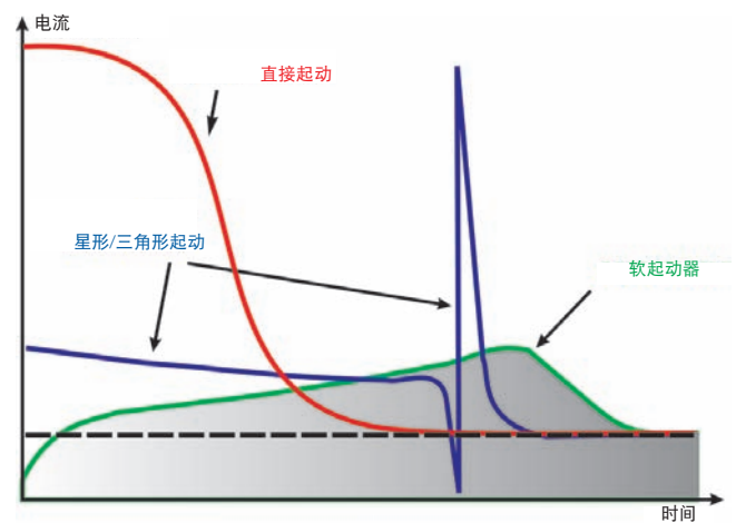
电机起动方法比较
