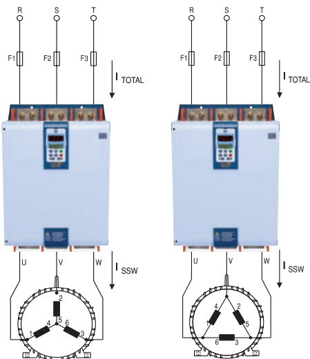
SSW-06外接
